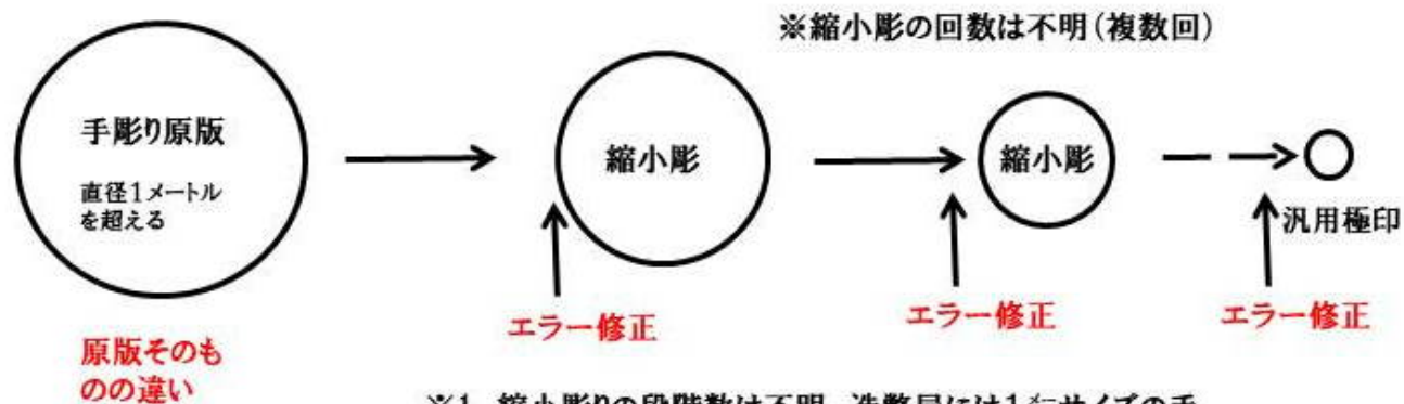
図1) 極印の製作手順(概念図)
